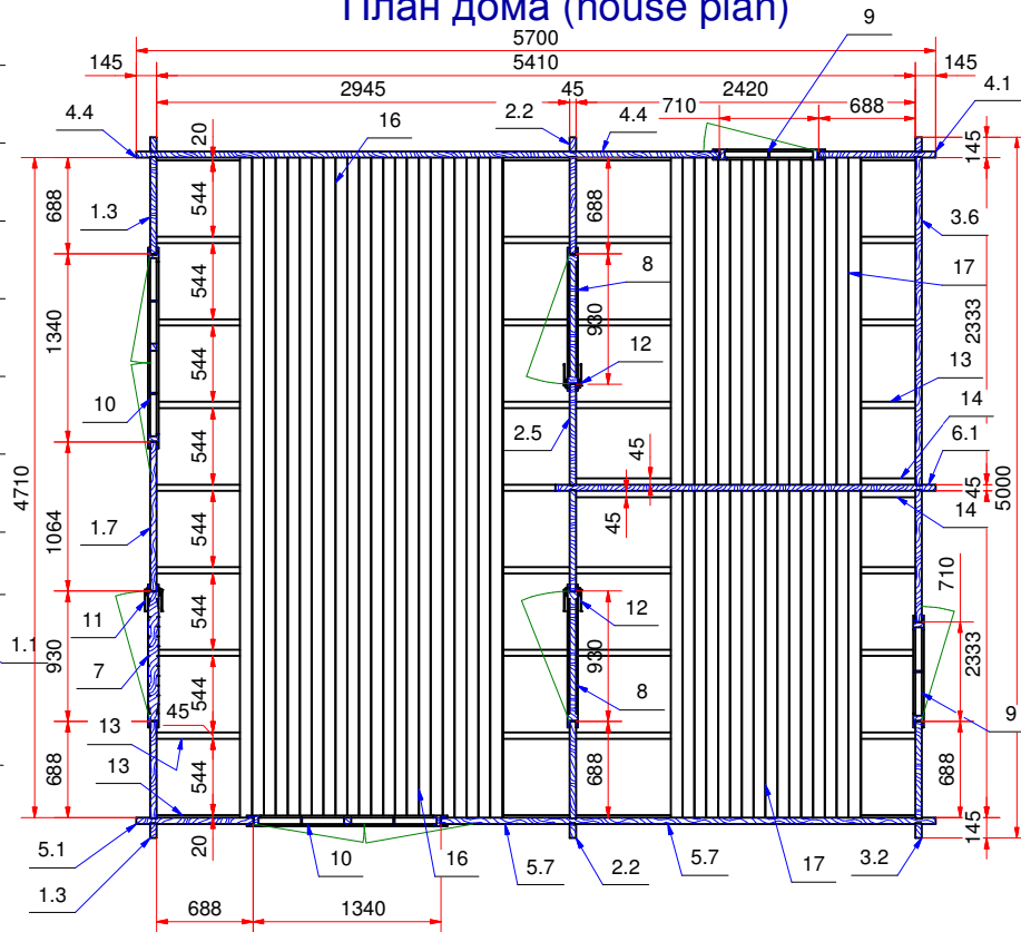
План дома (house plan)
